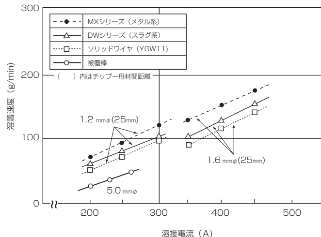
図1 溶着速度の一例
