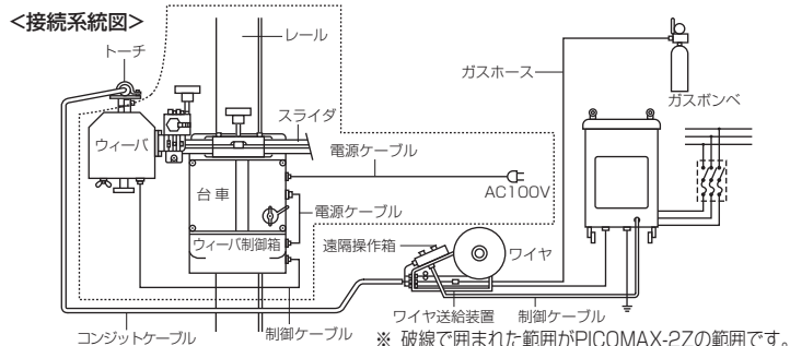
(横向片面溶接例)
