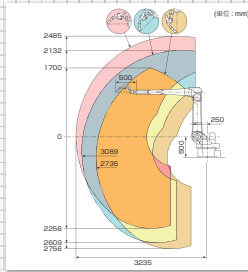
大型溶接ロボット： ARCMAN™ A80
