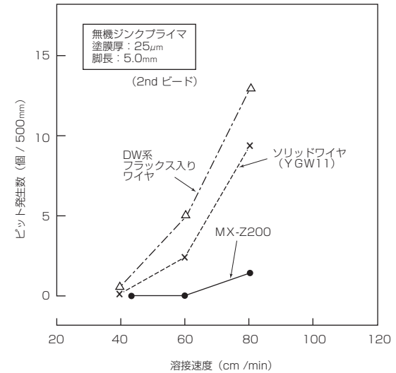
図3 耐プライマ性の一例
