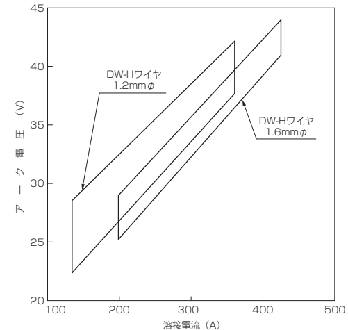
図2 電流・電圧の適正範囲（DW-Hワイヤ）
