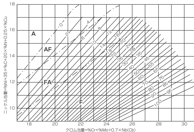
JIS Z 3119の組織図C (WRC-1992線図に同等)
