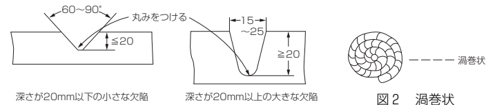
図1 開先形状
