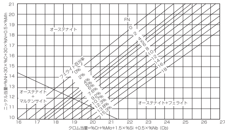
JIS Z 3119の組織図B (ディロングの組織図に同等)
