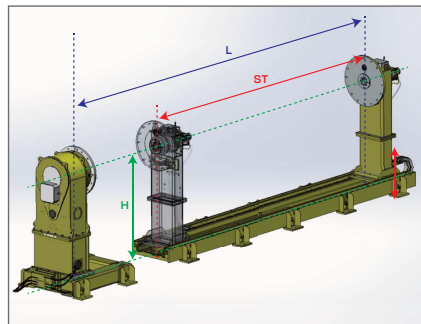
■R1-1500EL(1500kg仕様) 寸法組合せ一覧 (単位:mm)
