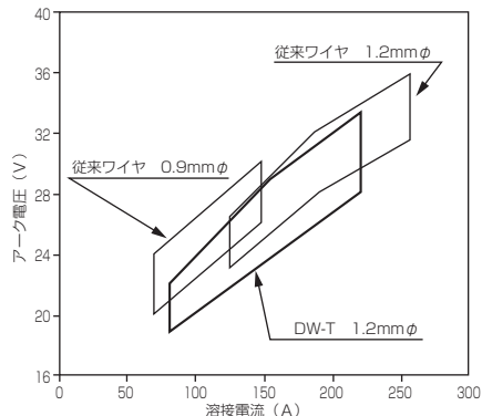
図1 適正電流・電圧範囲 (CO 2 、下向き)
