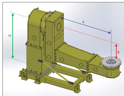
■K2-500EL(500kg仕様) 寸法組合せ一覧 (単位:mm)
